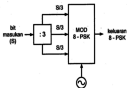
Gambar 1. Diagram blok pembangkitan sinyal 8-PSK
