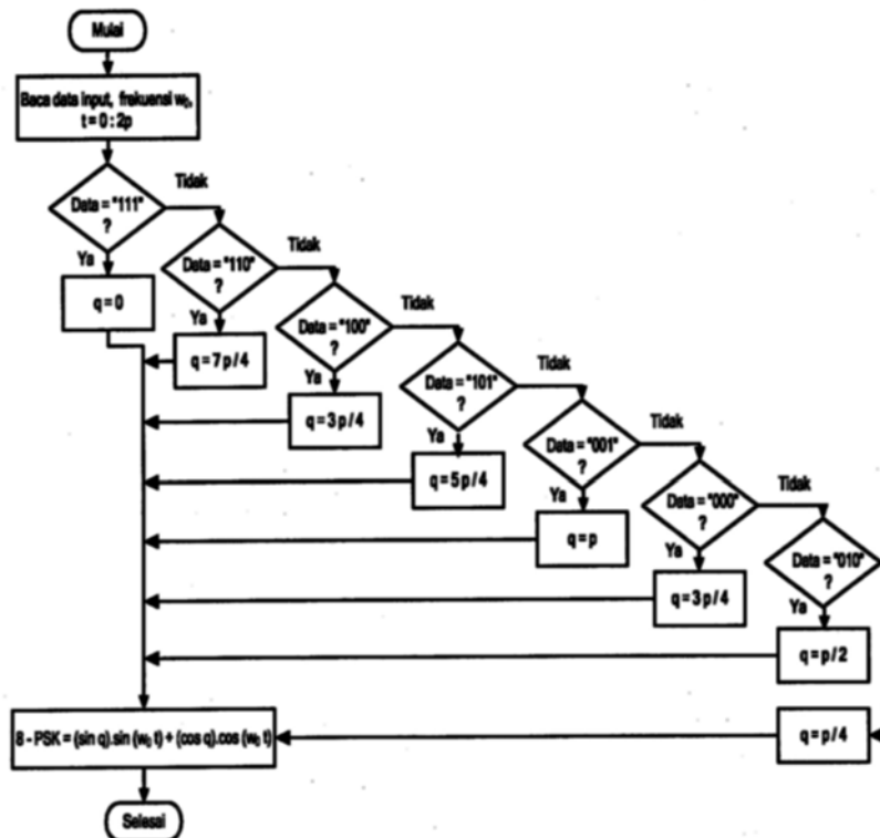
Gambar 3. Diagram alir simulasi pembangkitan sinyal 8-PSK
